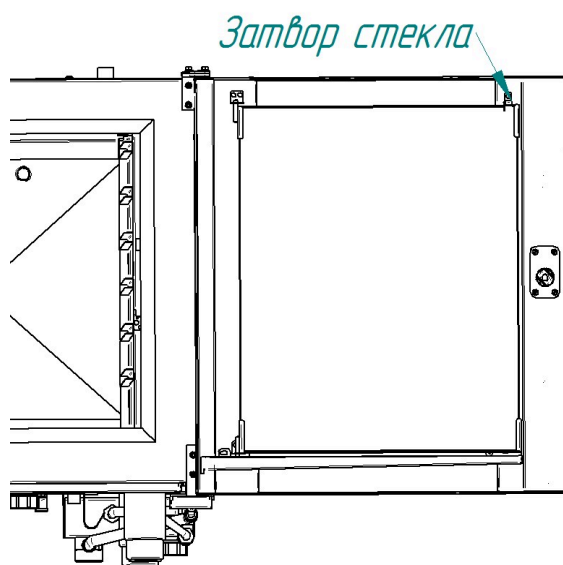
Рис.6 Месторасположение затвора внутреннего стекла двери
